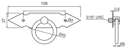
Cód. 530 - Puxador Anel 45mm 3/16 Espelho Retangular - Pintado Preto Cód. 531 - Puxador Anel 45mm 3/16 Espelho Retangular - Ouro Velho
