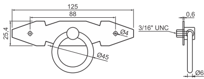
Cód. 526 - Puxador Anel 45mm 3/16 Espelho Quadrado - Pintado Preto Cód. 527 - Puxador Anel 45mm 3/16 Espelho Quadrado - Ouro Velho
