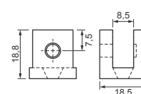
Cód. 1186 - Suporte U Plástico para Vidro 4mm - Branco Cód. 1187 - Suporte U Plástico para Vidro 4mm - Preto Cód. 1188 - Suporte U Plástico para Vidro 4mm - Cromado Cód. 1189 - Suporte U Plástico para Vidro 4mm - Dourado
