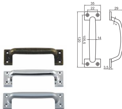
Cód. 520 - Puxador Alça 120mm - Cromado Cód. 521 - Puxador Alça 120mm - Ouro Velho Cód. 807 - Puxador Alça 120mm - Prata Fosco
