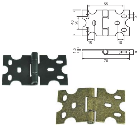
Cód. 1071 - Dobradiça Colonial Quadrada - Pintada Preta Cód. 1072 - Dobradiça Colonial Quadrada - Ouro Velho
