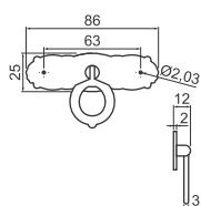
Cód. 1708 - Puxador Meia Lua Fino M4 - Ouro Velho
