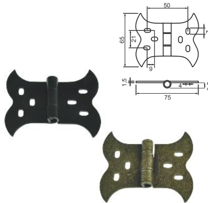
Cód. 1073 - Dobradiça Colonial Ponta - Pintada Preta Cód. 1074 - Dobradiça Colonial Ponta - Ouro Velho
