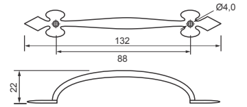
Cód. 1704 - Puxador Gaveta M4 Espelho Losango - Pintado Preto Cód. 1705 - Puxador Gaveta M4 Espelho Losango - Ouro Velho
