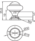
Cód. 1712 - Puxador Anel 35mm 3/16 Espelho Redondo - Pintado Preto Cód. 1711 - Puxador Anel 35mm 3/16 Espelho Redondo - Ouro Velho
