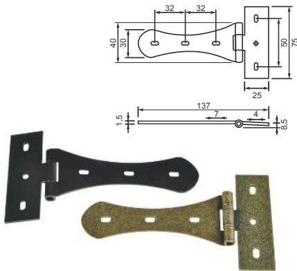
Cód. 1077 - Dobradiça Colonial Gota - Pintada Preta Cód. 1078 - Dobradiça Colonial Gota - Ouro Velho
