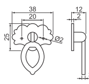
Cód. 1707 - Puxador Meia Lua Pequeno Estriado - Ouro Velho
