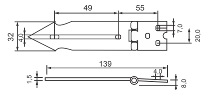
Cód. 1075 - Dobradiça Colonial Lança - Pintada Preta Cód. 1076 - Dobradiça Colonial Lança - Ouro Velho
