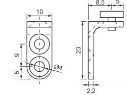
Cód. 780 - Suporte Prat. Zamac Leve 13,5 x 13,5mm 2 Furos - Niquelado Cód. 781 - Suporte Prat. Zamac Leve 13,5 x 13,5mm 2 Furos - Pintado Branco Cód. 782 - Suporte Prat. Zamac Leve 13,5 x 13,5mm 2 Furos - Cromado Cód. 783 - Suporte Prat. Zamac Leve 13,5 x 13,5mm 2 Furos - Zincado Branco Cód. 951 - Suporte Prat. Zamac Leve 13,5 x 13,5mm 2 Furos - Pintado Preto Cód. 1353 - Suporte Prat. Zamac Super Leve 13,5 x 13,5mm 2 Furos - Niquelado Cód. 1354 - Suporte Prat. Zamac Super Leve 13,5 x 13,5mm 2 Furos - Pint. Branco Cód. 1355 - Suporte Prat. Zamac Super Leve 13,5 x 13,5mm 2 Furos - Cromado Cód. 1356 - Suporte Prat. Zamac Super Leve 13,5 x 13,5mm 2 Furos - Zinc. Branco
