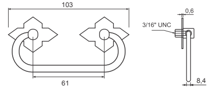
Cód. 1702 - Puxador Porta M4 Espelho Losango - Pintado Preto Cód. 1703 - Puxador Porta M4 Espelho Losango - Ouro Velho
