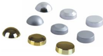
Cód. 580 - Acabamento Rosca Int. 19mm Chato Zamac - Cromado Cód. 581 - Acabamento Rosca Int. 19mm Chanfrado Zamac - Cromado Cód. 582 - Acabamento Rosca Int. 19mm Redondo Zamac - Cromado Cód. 801 - Acabamento Rosca Int. 19mm Chato Zamac - Prata Fosco Cód. 802 - Acabamento Rosca Int. 19mm Chanfrado Zamac - Prata Fosco Cód. 803 - Acabamento Rosca Int. 19mm Redondo Zamac - Prata Fosco Cód. 1211 - Acabamento Rosca Int. 19mm Chato Zamac - Dourado Cód. 1212 - Acabamento Rosca Int. 19mm Chanfrado Zamac - Dourado Cód. 1213 - Acabamento Rosca Int. 19mm Redondo Zamac - Dourado
