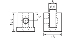
Cód. 583 - Botão Francês 19mm Zamac Estriado - Cromado Cód. 804 - Botão Francês 19mm Zamac Estriado - Prata Fosco Cód. 1214 - Botão Francês 19mm Zamac Estriado - Dourado Cód. 809 - Botão Francês 19mm Zamac Liso - Cromado Cód. 810 - Botão Francês 19mm Zamac Liso - Prata Fosco Cód. 1215 - Botão Francês 19mm Zamac Liso - Dourado
